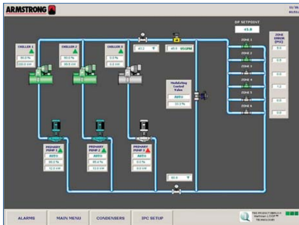
Pantalla general de la planta enfriada por agua
