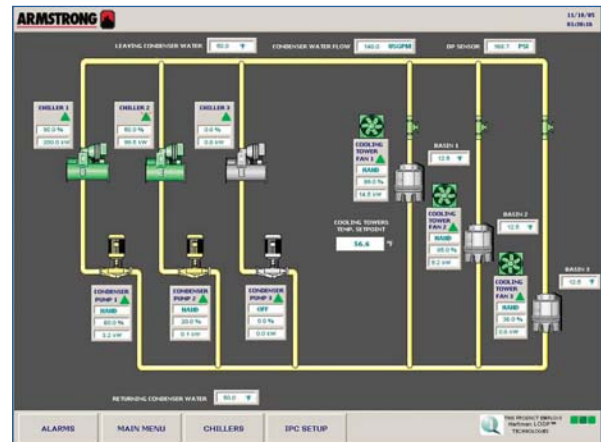
Pantalla del circuito de agua del condensador
