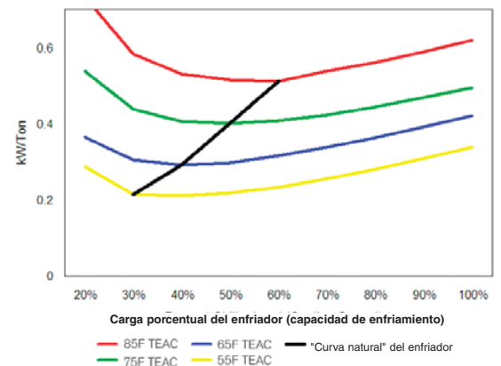
TEAC - Temperatura de entrada del agua del condensador
