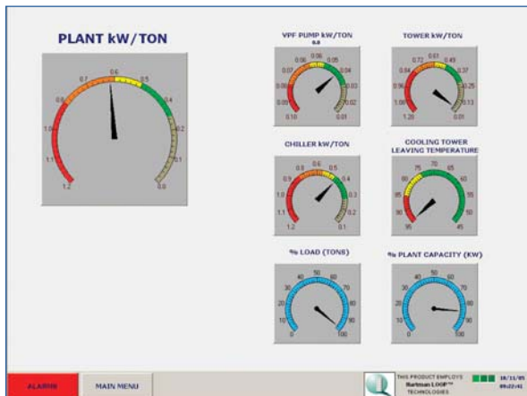
Pantalla de medición del desempeño de la planta
