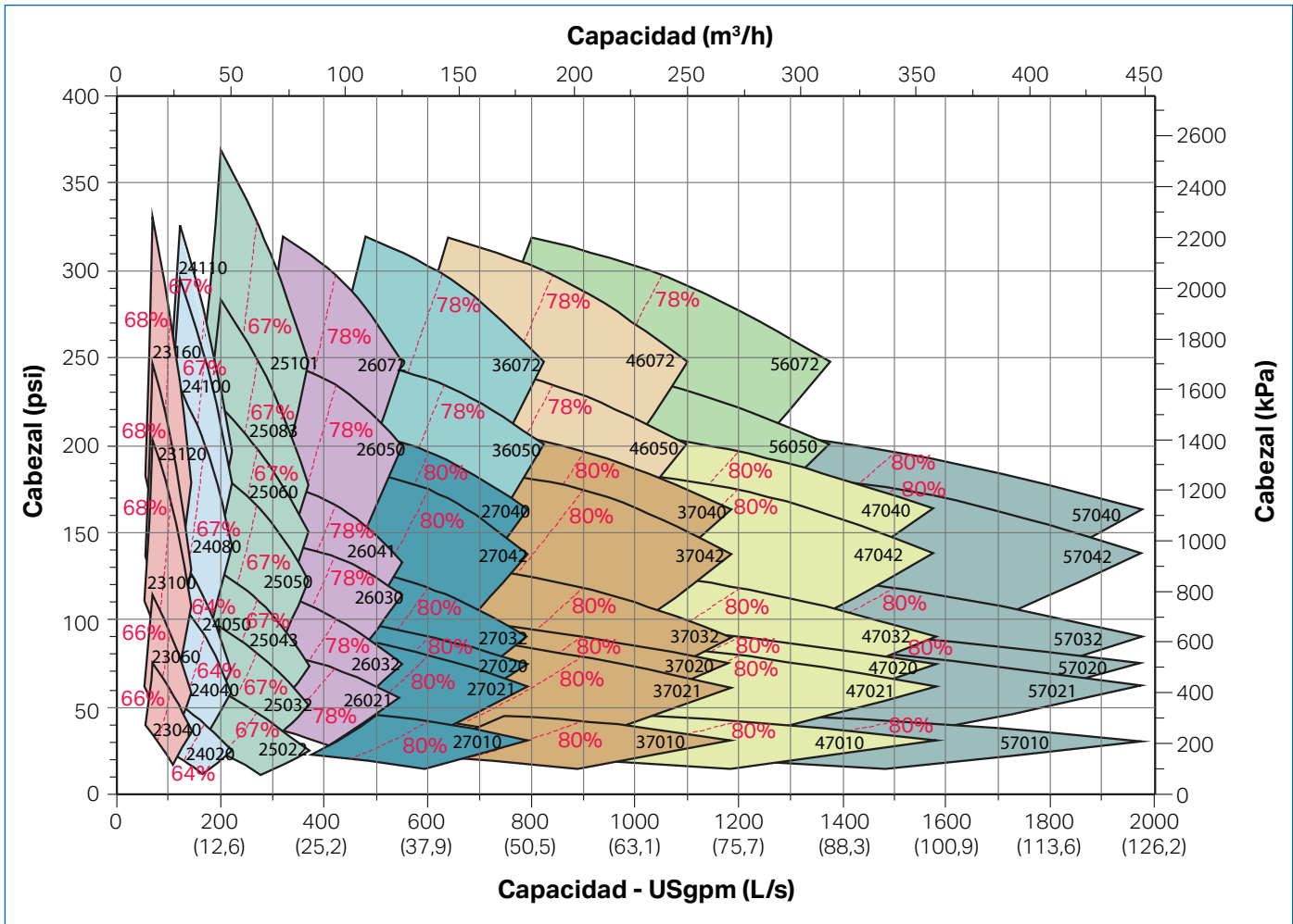
Sistema impulsor Serie 6800 IVS con diseño compacto
